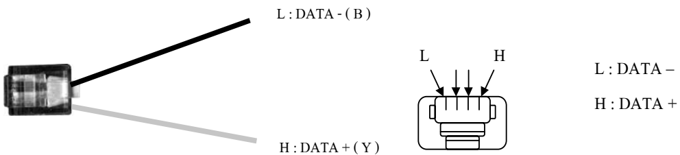
รูปที่ 10.4 แสดงการเข้าสายของเครื่อง V-PHONE
