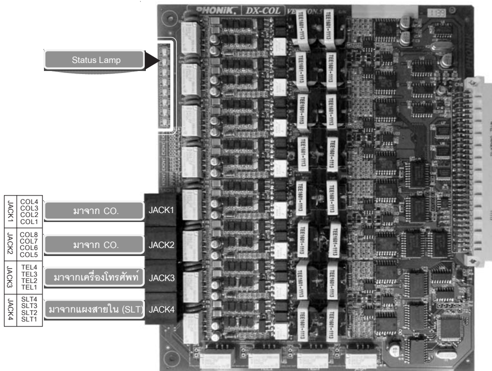
รูปที่ 4.4 แสดงการวางอุปกรณ์ของแผง DX-8COL/C.V5
