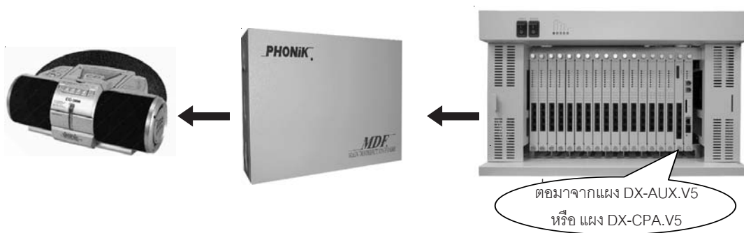
รูปที่ 7.5 แสดงการต่อ External Music
